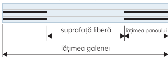
DISPOZIȚIE ÎN POZIȚIA STRÂNSĂ
