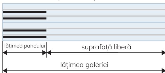
DISPOZIȚIE ÎN POZIȚIA STRÂNSĂ
