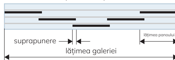
DISPOZIȚIE ÎN POZIȚIA EXTINSĂ
