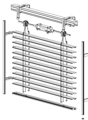
Jaluzea exterioară Z90 - motor Schema de bază
