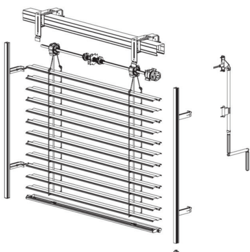
Jaluzea exterioară Z90 - manivelă Schema de bază
