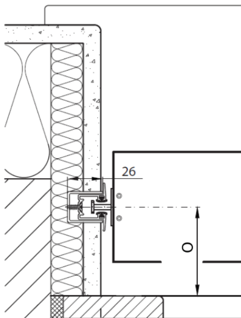
Montajul ghidajului lateral VL7 cu carcasă încastrată ZP
