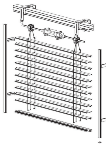
Jaluzea exterioră Z70 - motor Schema de bază
