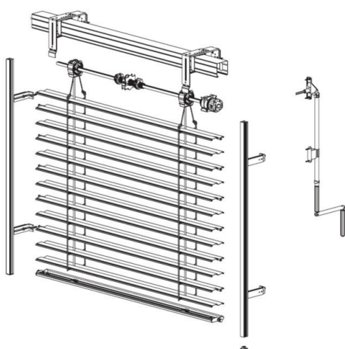
Jaluza exterioră S90 - manivelă Schema de bază
