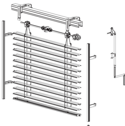
Jaluzea exterioară C80 - manivelă Schema de bază
